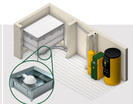
KWB PELLET BOX AVEC TRANSPORT PAR ASPIRATION
