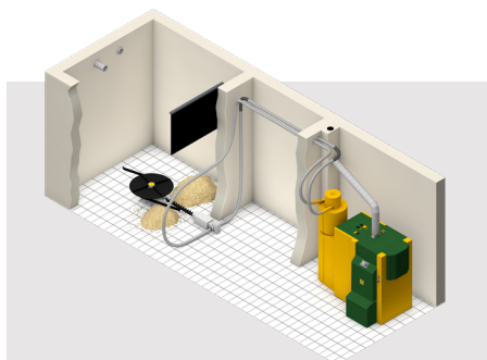
DESSILEUR À GRANULÉS KWB PLUS AVEC TRANSPORT PAR ASPIRATION
