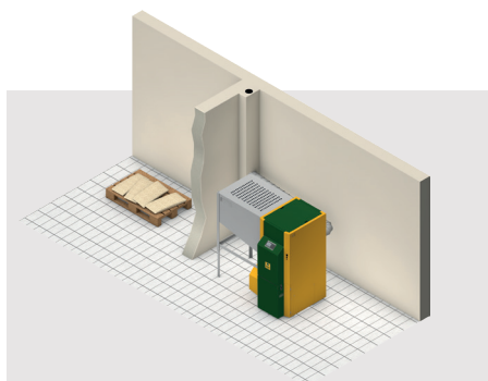
RÉSERVOIRS DE STOCKAGE KWB 300 L
