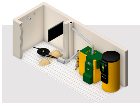
DESSILEUR À GRANULÉS PLUS À VIS COUDÉE
