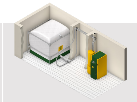
KWB BIG BAG À GRANULÉS AVEC TRANSPORT PAR ASPIRATION
