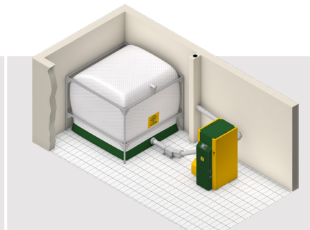
KWB BIG BAG À GRANULÉS À VIS COUDÉE
